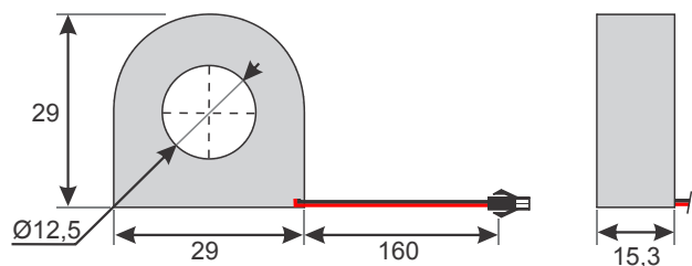
Transformador de corrente (TC)
